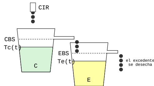
FIGURA 16.12: Algoritmo de cubo de tokens de tipo srTCM
